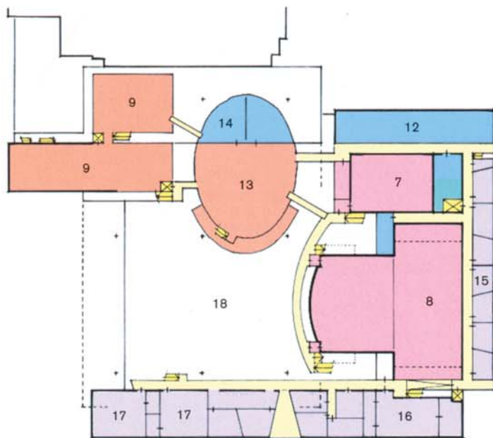
Eerste verdieping
