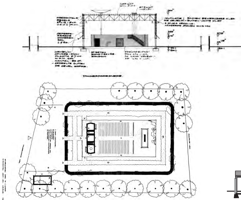
Ludgerkerk, doorsnede en plattegrond/ Ludger Church, section en floor plan
